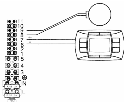
Датчик уличной температуры
